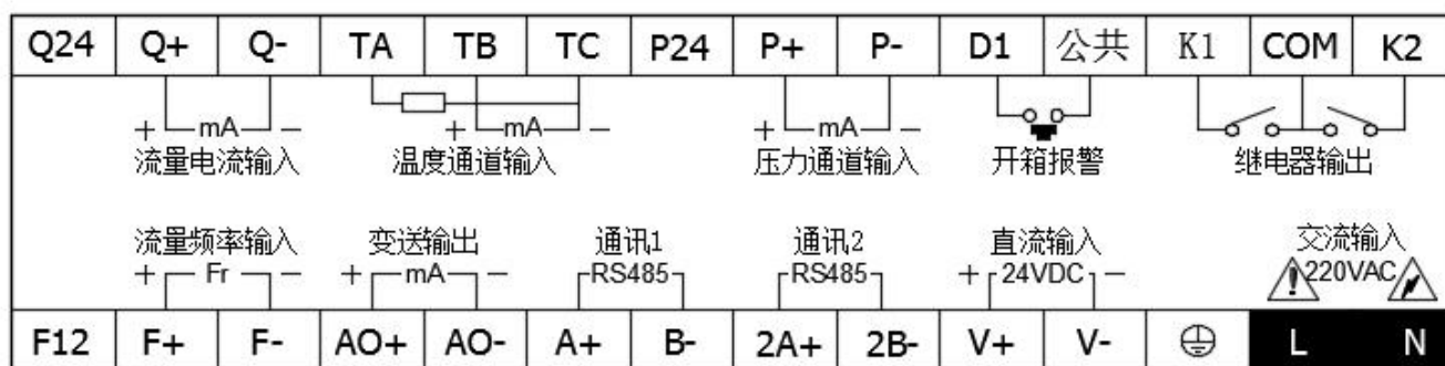
双电源接线图
