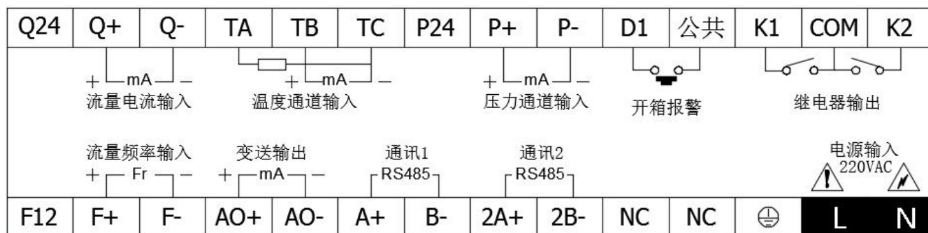
单电源接线图
