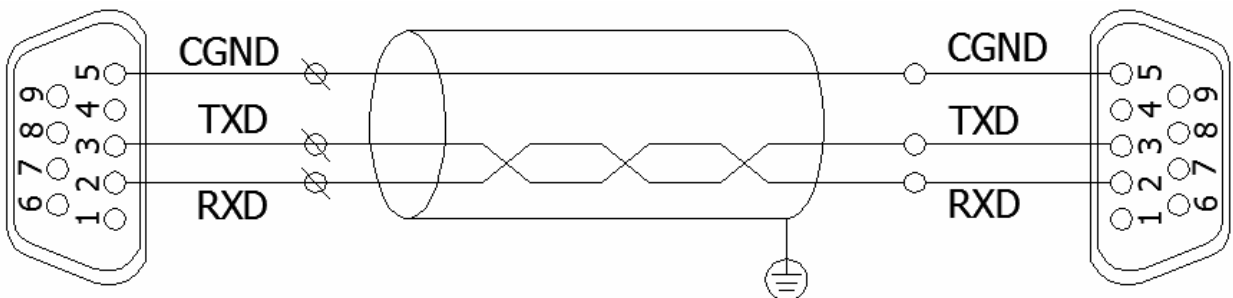
仪表侧RS232C通讯接口
